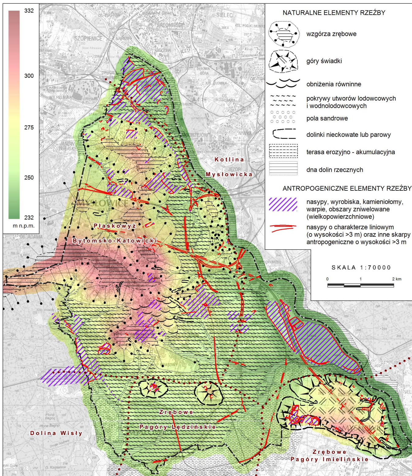
Ryc.3 Rzeźba terenu
