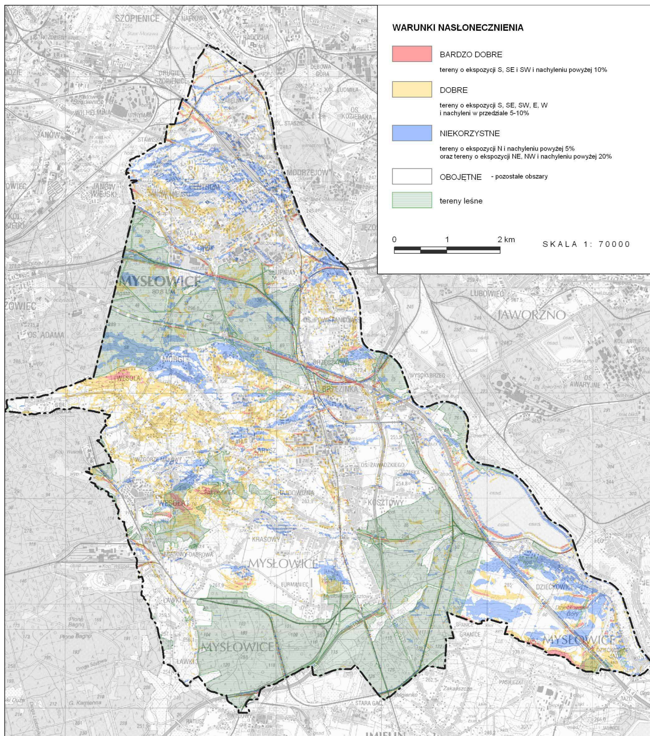
Ryc. 7. Nasłonecznienie terenu
