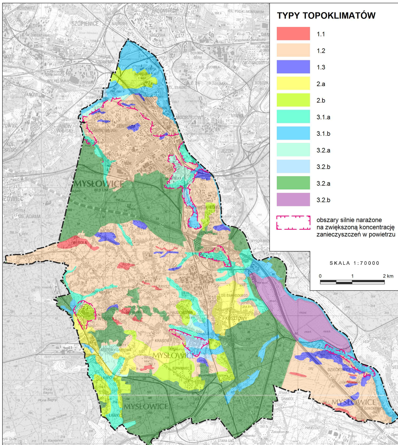
Ryc.5. Warunki topoklimatyczne
