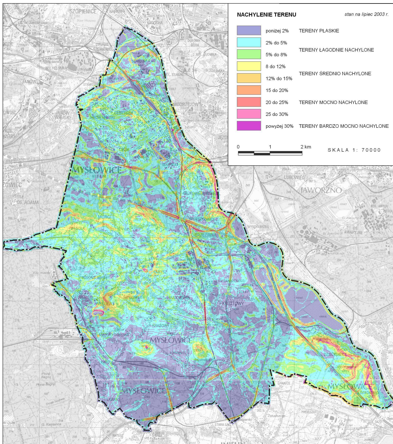
Ryc.4 Nachylenia terenu
