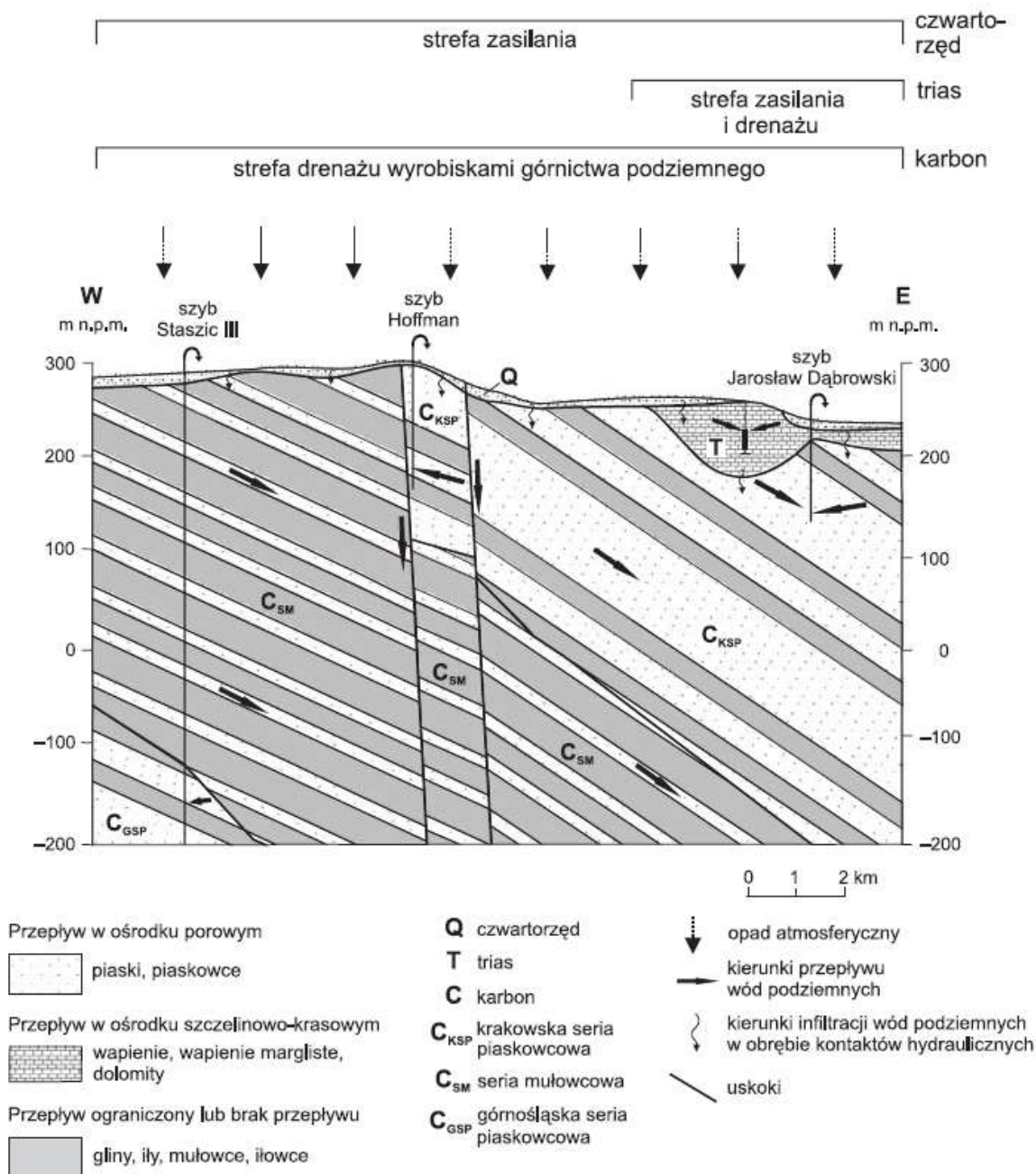
Ryc. 2. Przekrój hydrogeologiczny i schemat krążenia wód podziemnych w profilu pionowym w południowej części Myśłowic
