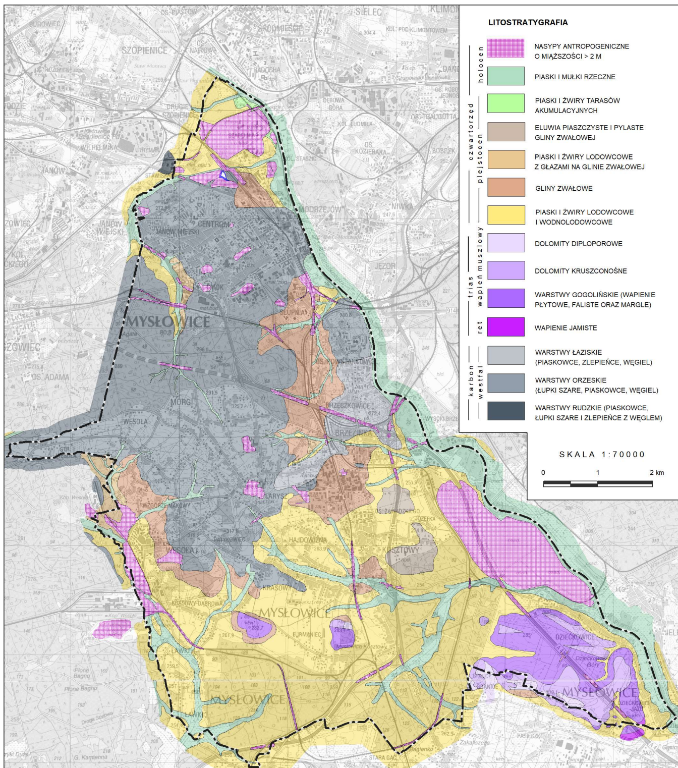
Ryc.1 Budowa geologiczna
